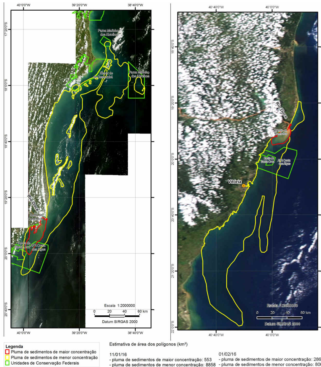
Figura 3: Mapas de satélite da pluma de sedimentos em 11/01/2016 (esq.) e 01/02/2016 (dir.). Fonte: adaptado de mapas elaborados por NUGEO/SP - IBAMA, a partir de imagens de satélite SPOT 6 e 7/NAOMI - AIRBUS (11/01/2016) e AQUA/MODIS - NASA/Worldview (01/02/2016)
