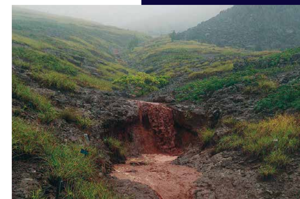
Figura 27: Córrego intermitente em período de chuva, transportando areia e sedimentos mais finos, como silte e argila.
