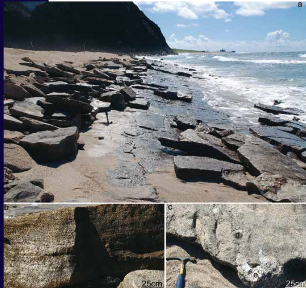
Figura 18: (a) Arenito na Praia das Tartarugas com proeminente laminação plano-paralela e inclinação de 13°, característica de face praiçal. (b) Detalhe da laminação plano-paralela. (c) Detalhe do arenito com seixos compostos por rochas vulcânicas (d) e restos de recife de algas calcárias (e) que, datado do pelo método do rádio carbono, forneceu idade entre 700 e 550 anos, indicando a idade máxima possível do arenito.
